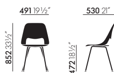
Jill Tube, Stahlrohruntergestell, nicht stapelbar,
